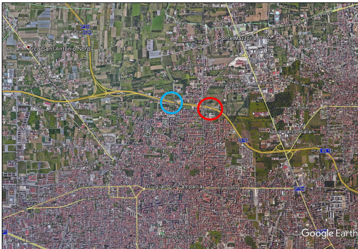
Fig. 3 – Posizionamento, rispetto al Centro Storico di Giugliano in Campania, dei nuovi svincoli da realizzare lungo la SS 162 NC “Asse Mediano”, in corrispondenza di Via Oasi del Sacro Cuore (in rosso) e di Via Santa Caterina da Siena (in azzurro).
