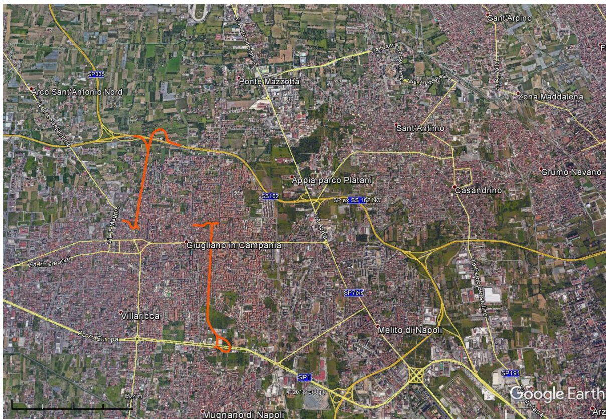
Fig. 2 – Posizionamento, rispetto al Centro Storico di Giugliano in Campania, di due nuove ipotesi di svincolo: Svincolo n.1: collegamento con la SS 162 NC “Asse Mediano”, con la realizzazione di una galleria bidirezionale (in arancione) volta a collegare tale svincolo con la viabilità comunale e, in particolare, con la Via Giulia e la Via Benedetto Croce; Svincolo n.2: collegamento della SPI “ex Circumvallazione Esterna di Napoli”, con la realizzazione di una galleria bi-direzionale, volta a collegare tale svincolo con la viabilità comunale e, in particolare, con la Via Fiardini e la Via Cumana.
